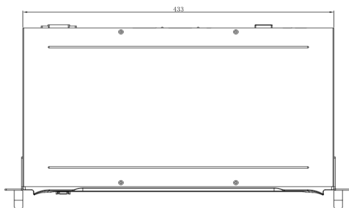
顶面板尺寸图
