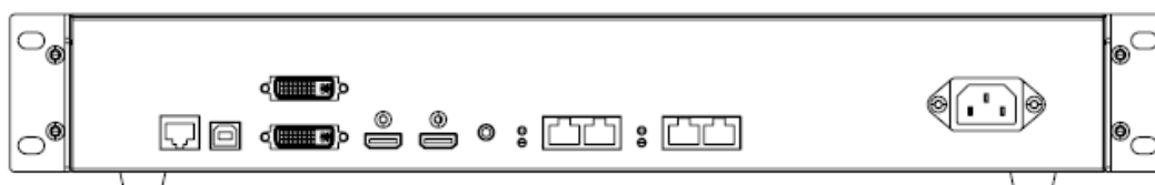
后面板尺寸图
