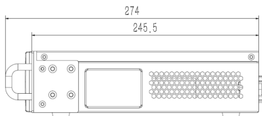
侧面板尺寸图
