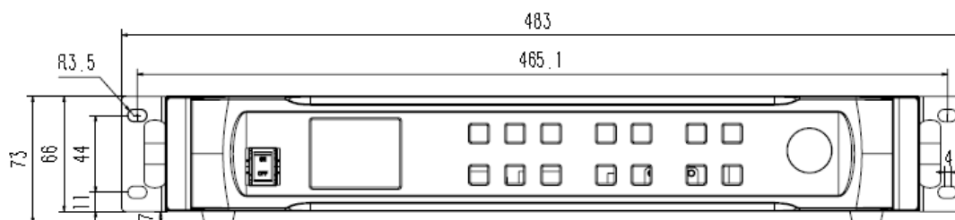
前面板尺寸图
