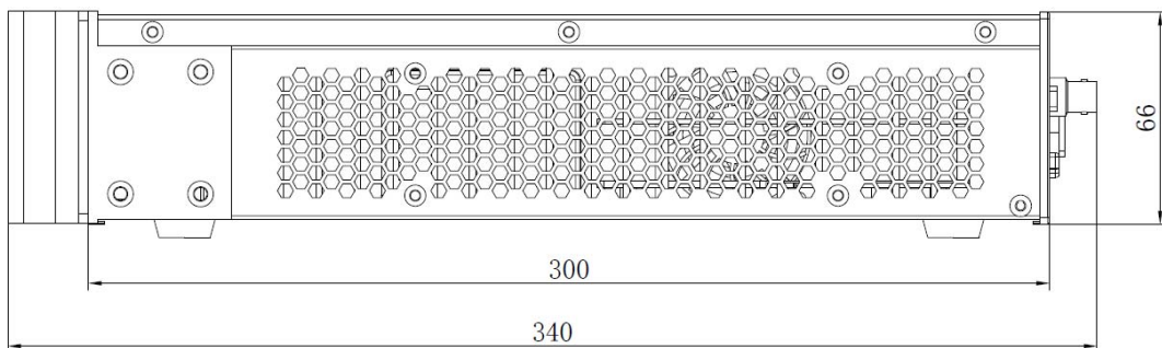
侧面尺寸图
