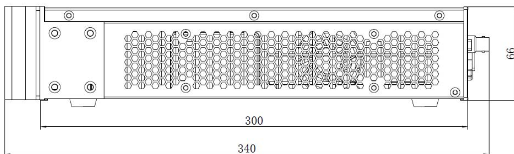
侧面尺寸图
