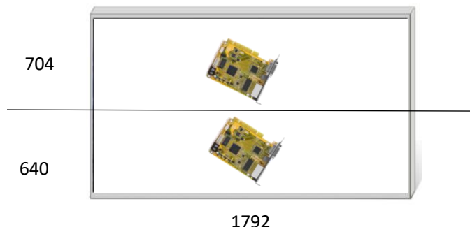
发送卡带载示意图
